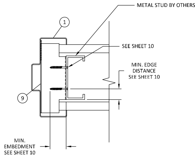
I 7 HORIZONTAL SECTION Z ANCHOR METAL STUD
